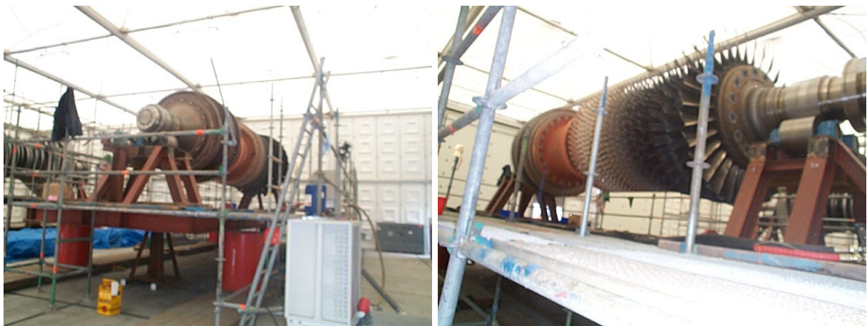
(overzicht turbinerotor voor het stralen)
